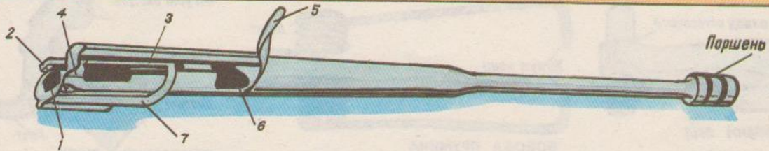
ЗАТВОРНА РАМА З ГАЗОВИМ ПОРШНЕМ
