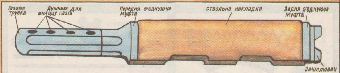
ГАЗОВА ТРУБКА ІЗ СТВОЛЬНОЮ НАКЛАДКОЮ
