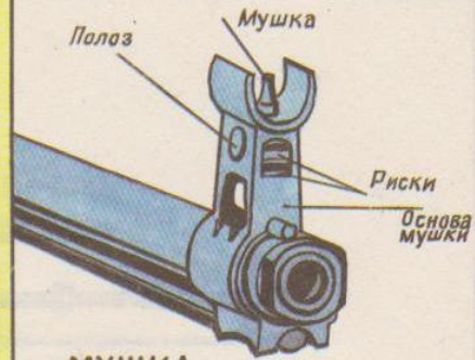
МУШКА
